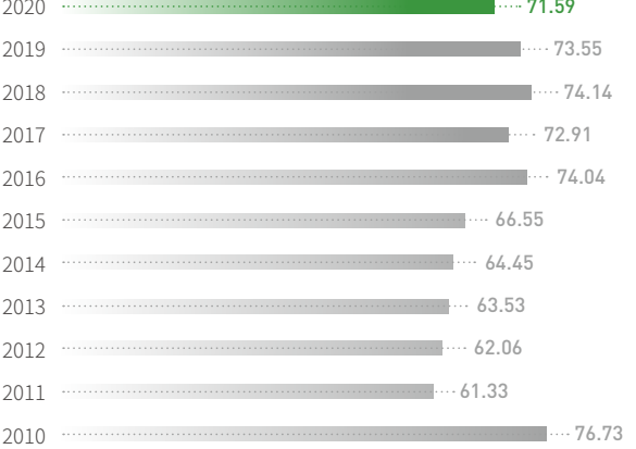
2010-2020 年吨水泥综合能耗 单位：千克标准煤 / 吨
