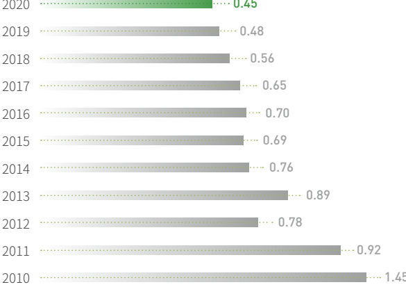
2010-2020 年吨水泥熟料氮氧化物排放量 单位：千克 / 吨
